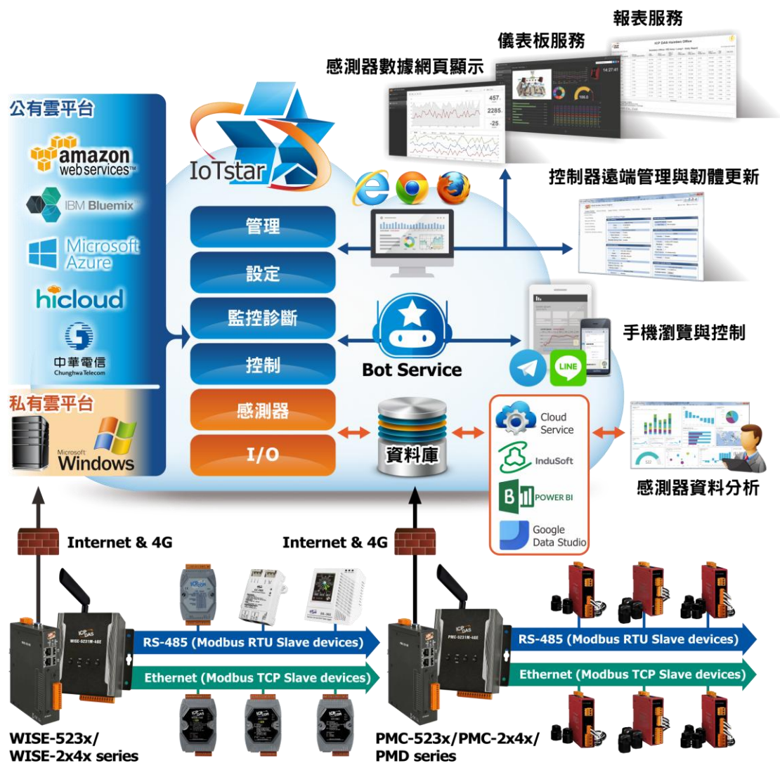
圖 1-1 IoTstar 系統架構圖
